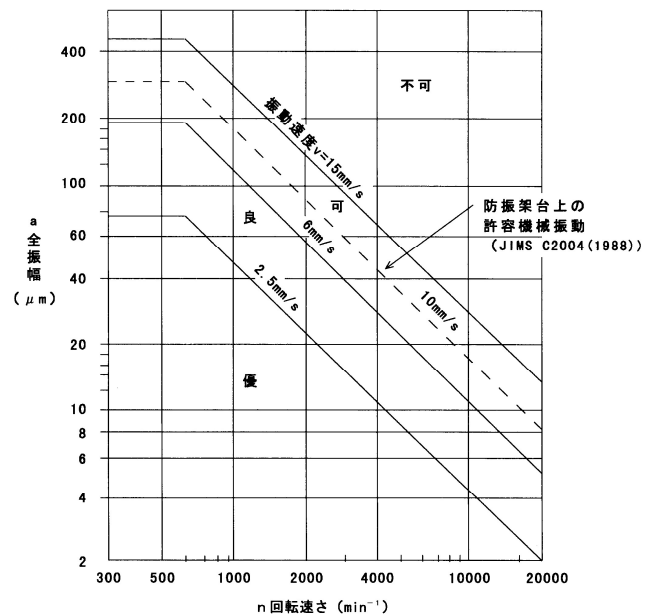
図 4.5.1 振動の許容値 (軸受箱上において)
